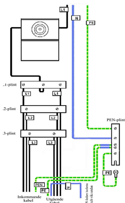
Illustration för 5-ledarkabel
