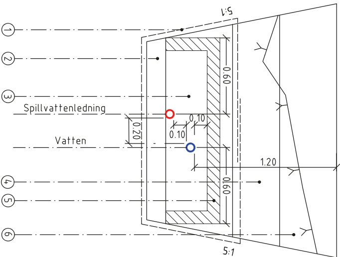
TYPSEKTION 1 SPILLVATTENLEDNING OCH VATTEN I BERGSCHAKT
