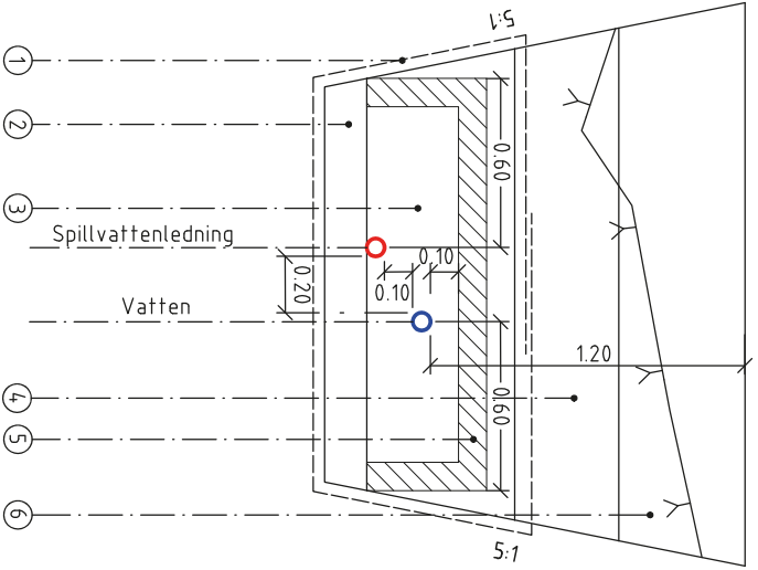
TYPESEKTION 1 SPILLVATTENLEDNING OCH VATTEN I BERGSCHAKT
