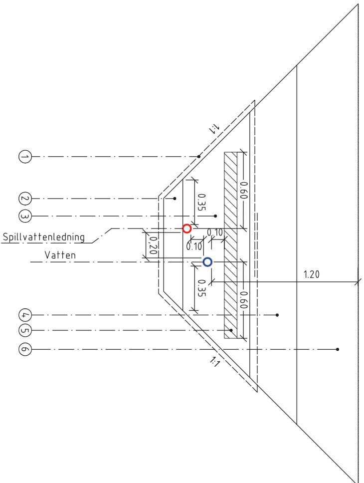
TYPESEKTION 2 SPILLVATTENLEDNING OCH VATTEN I JORDSCHAKT
