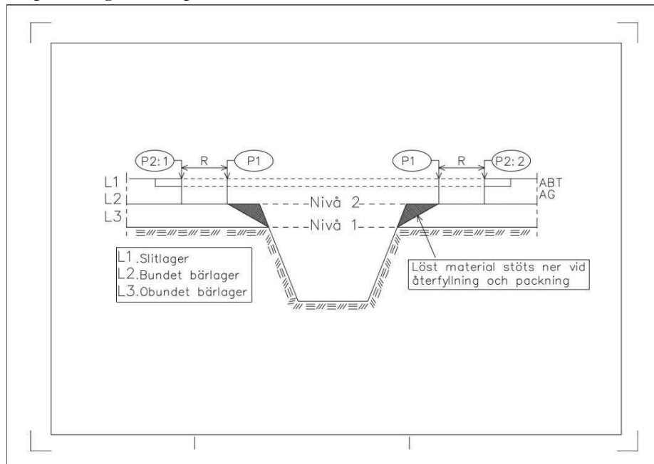
Figur 1. Tvärsektion på schakt
