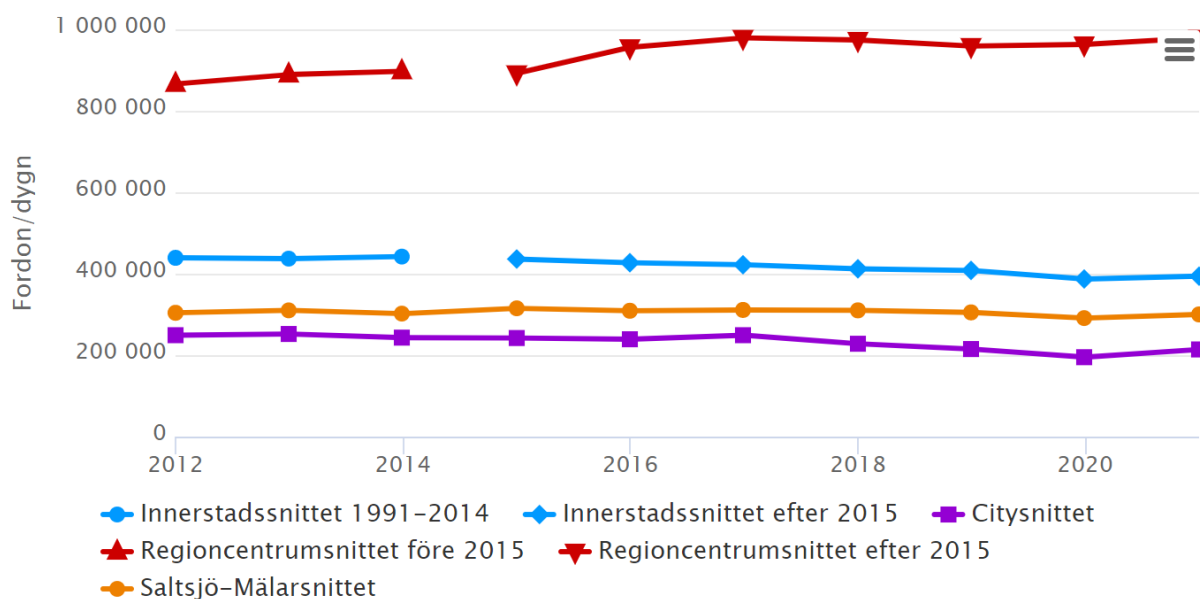
Figur 6. Antal fordonspassager per dygn i Stockholm.
